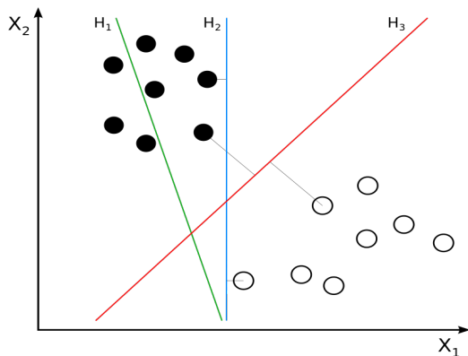
Hình 2. Mô phỏng thuật toán máy vector hỗ trợ.
